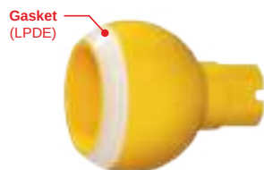
HGQ 2117 D5 Flat fan nozzle
